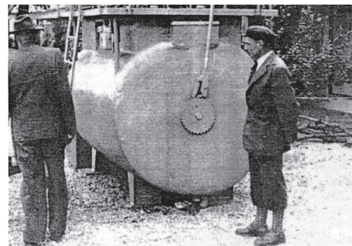
Bild 1: Kleinbiogasanlage für 10 GVE, System Hohenheim, auf einer landw. Ausstellung im Jahr 1956 Foto: Dr. Tietjen
